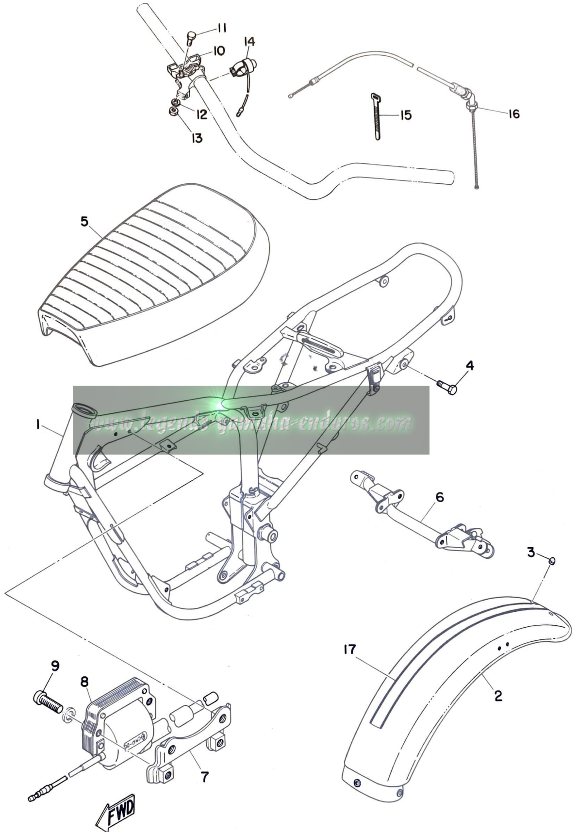
Fig. 7 FRAME · REAR FENDER · SEAT
