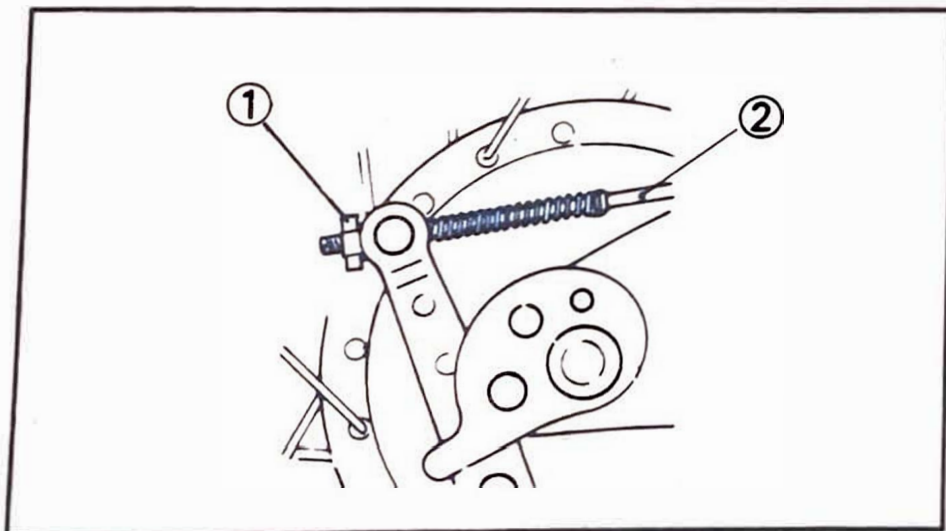
2. Brake rod
