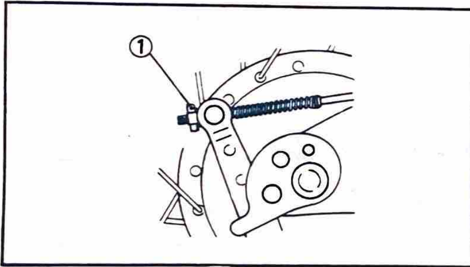
1. Adjuster
