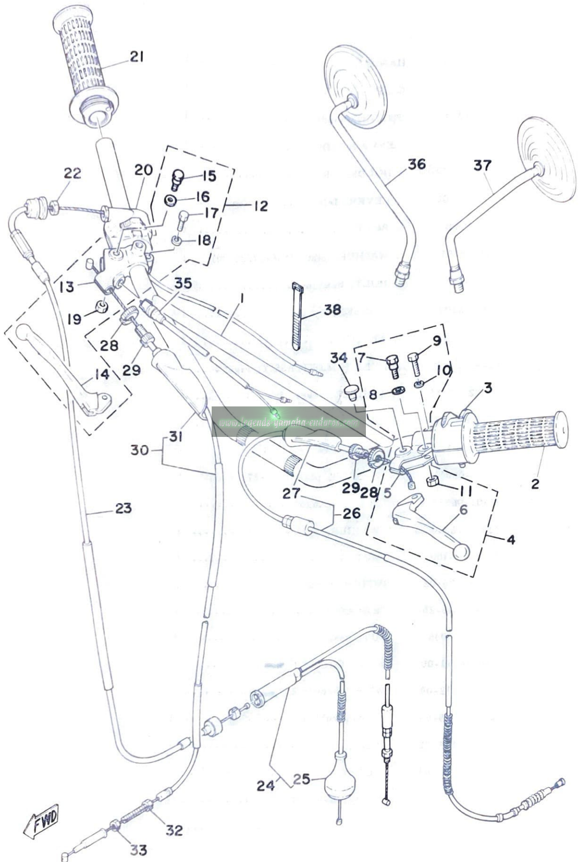
Fig. 20 HANDLE · WIRE
