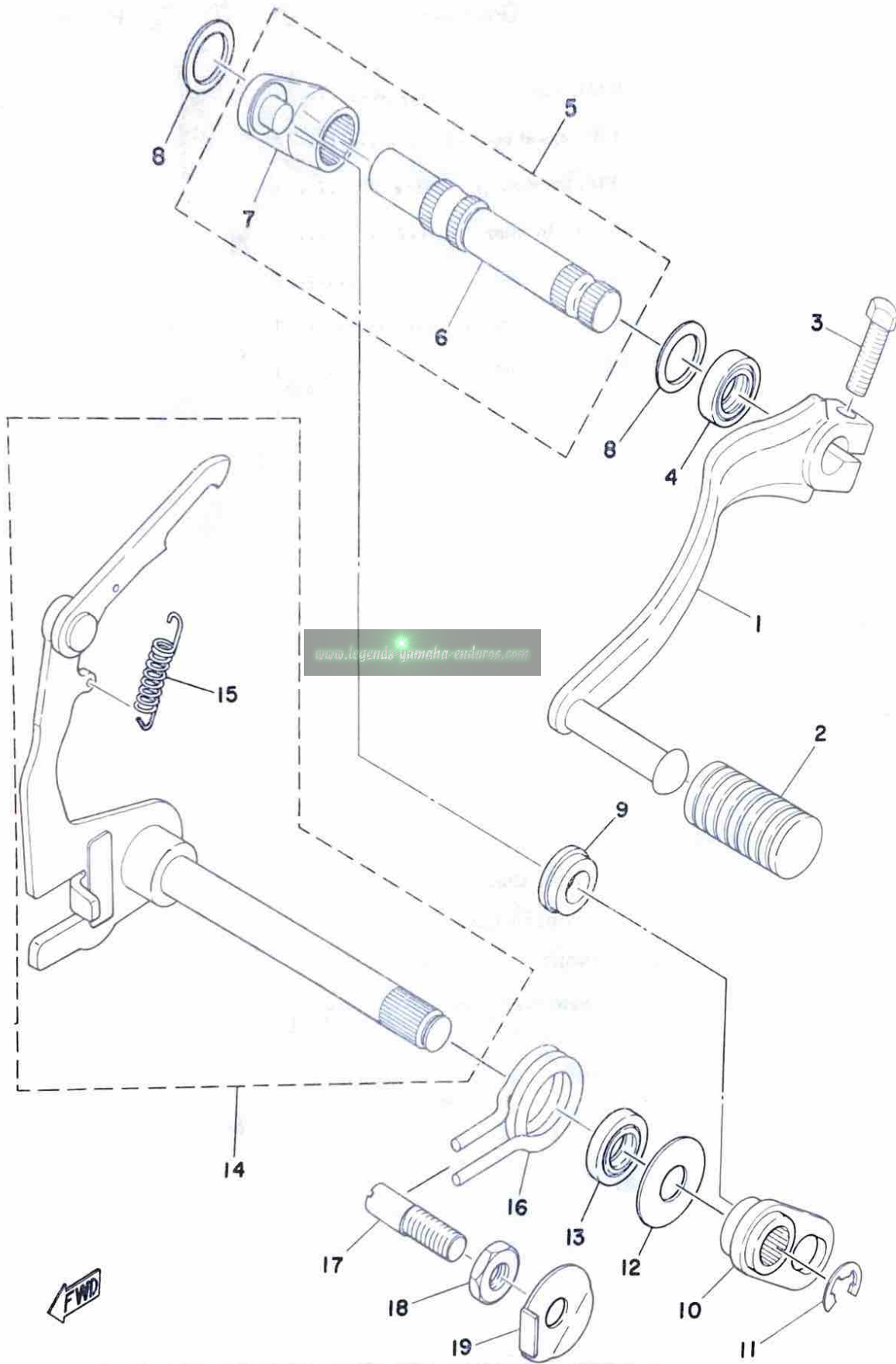
Fig.7 SHIFTER 2
