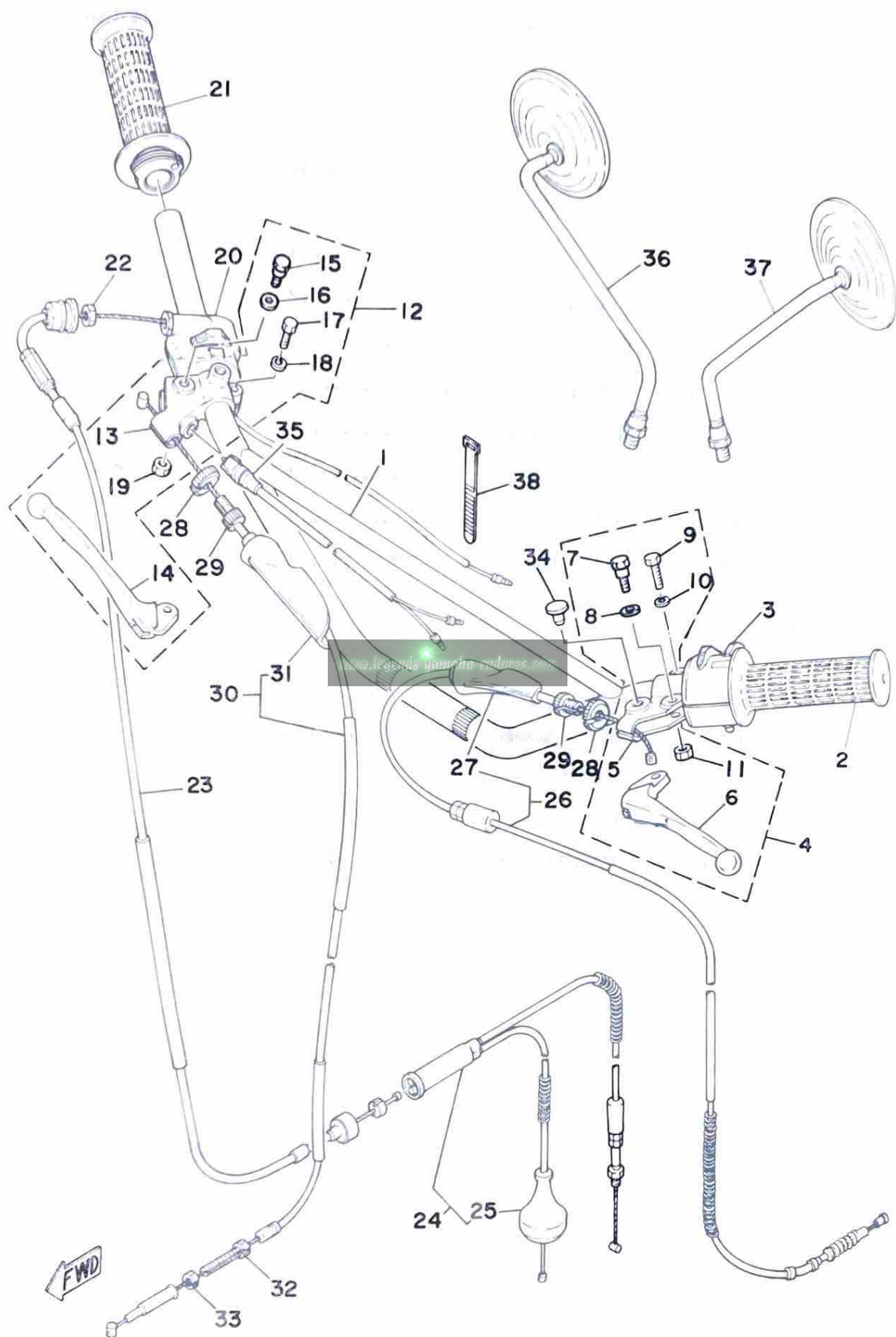
Fig. 20 HANDLE · WIRE
