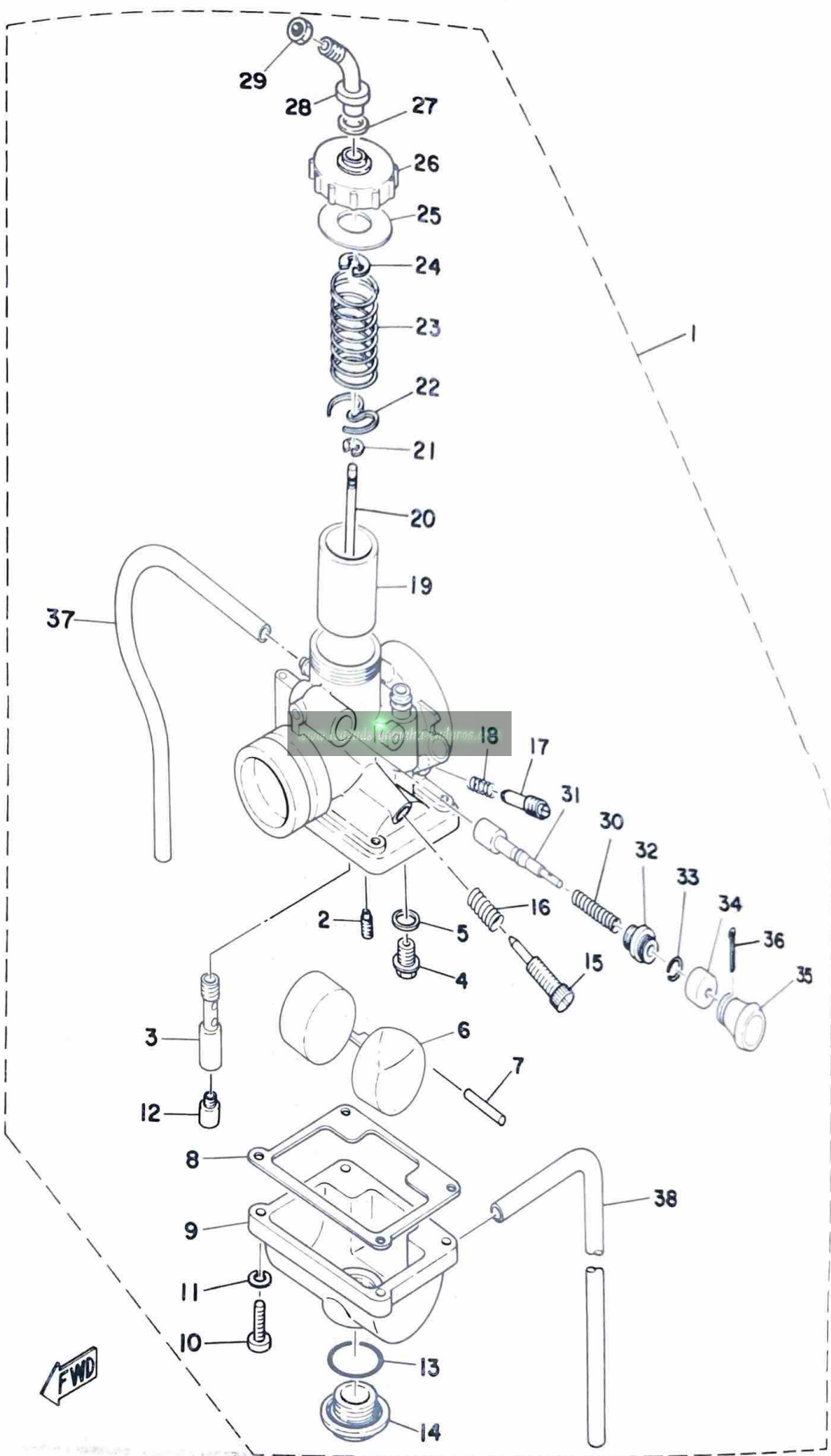
Fig. 10 CARBURETOR
