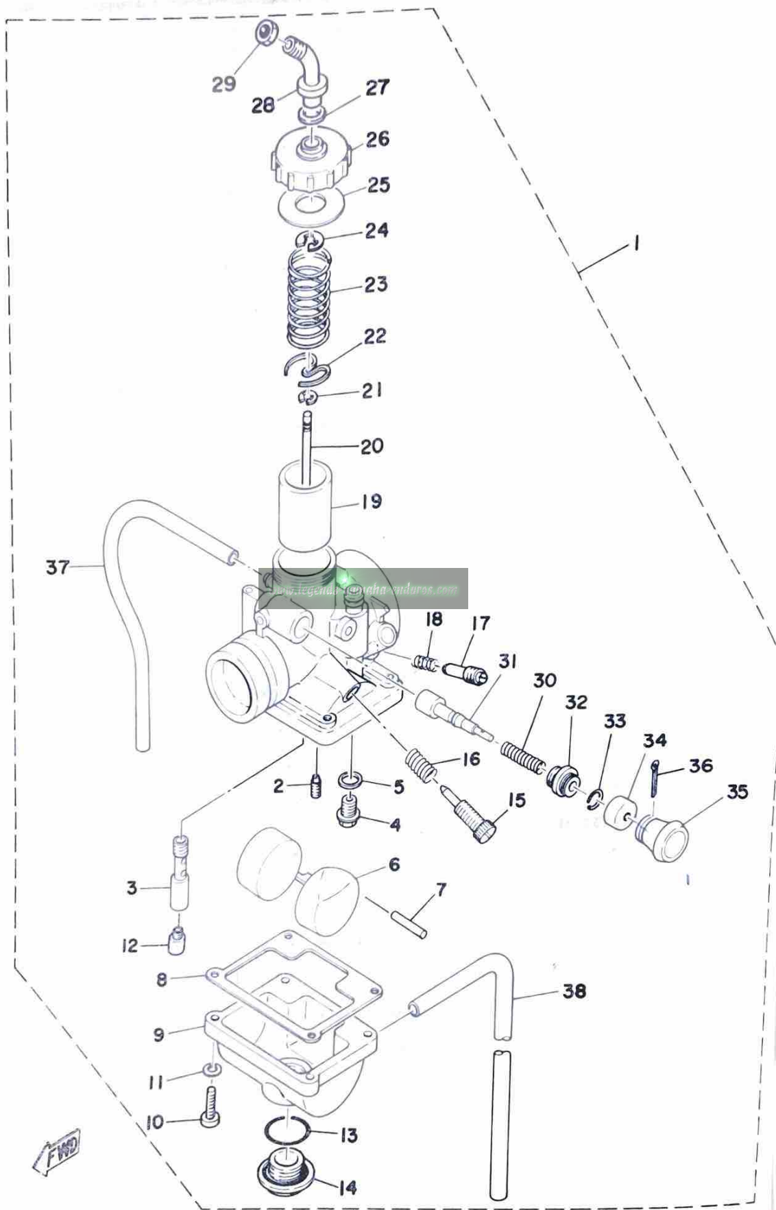
Fig. 10 CARBURETOR
