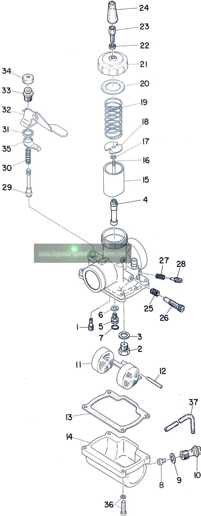
Fig. 4 CARBURETOR
