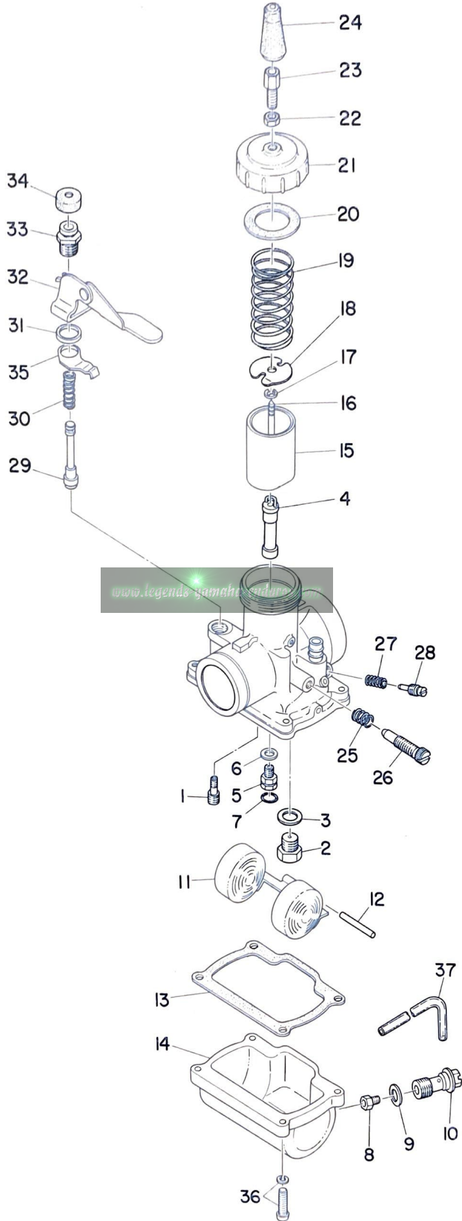
Fig. 4 CARBURETOR
