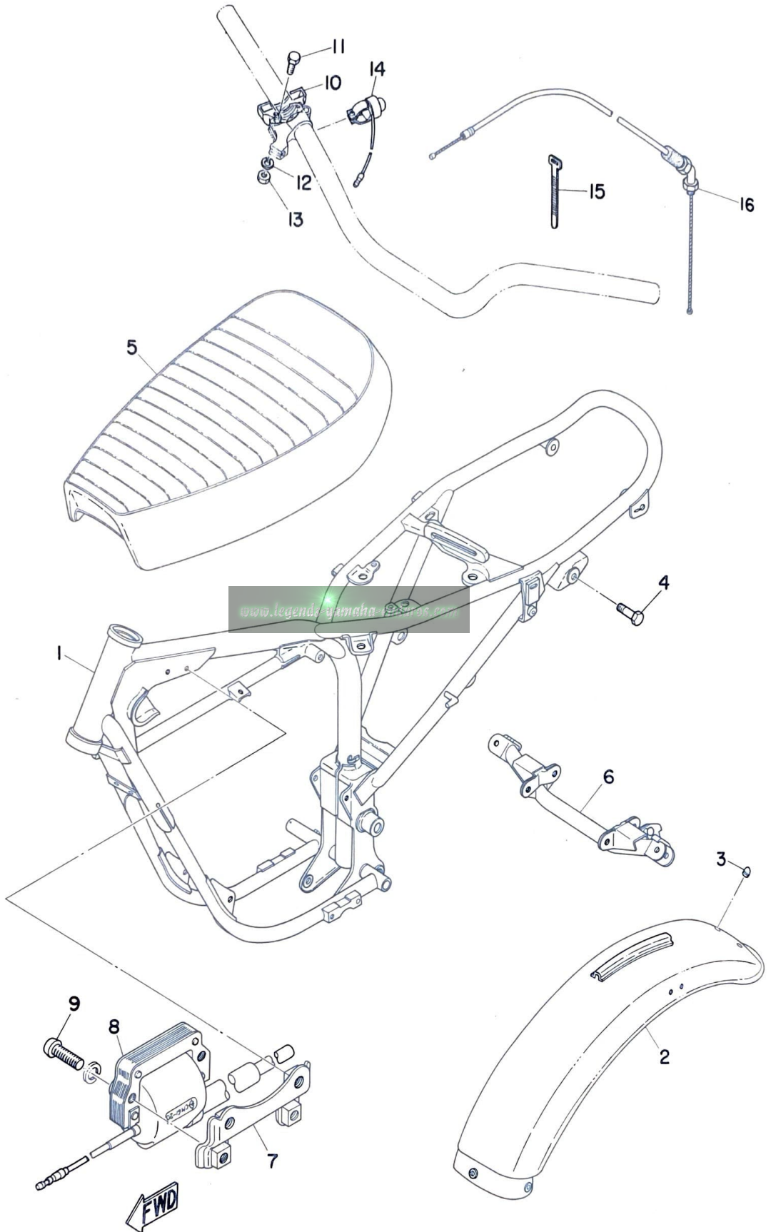
Fig. 6 FRAME · REAR FENDER · SEAT
