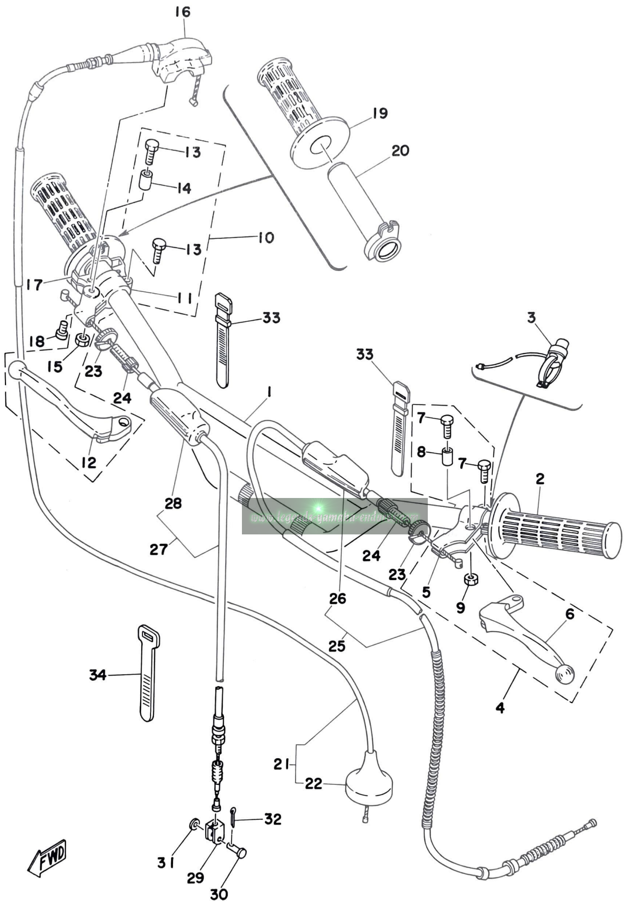
Fig. 19 HANDLE · WIRE
