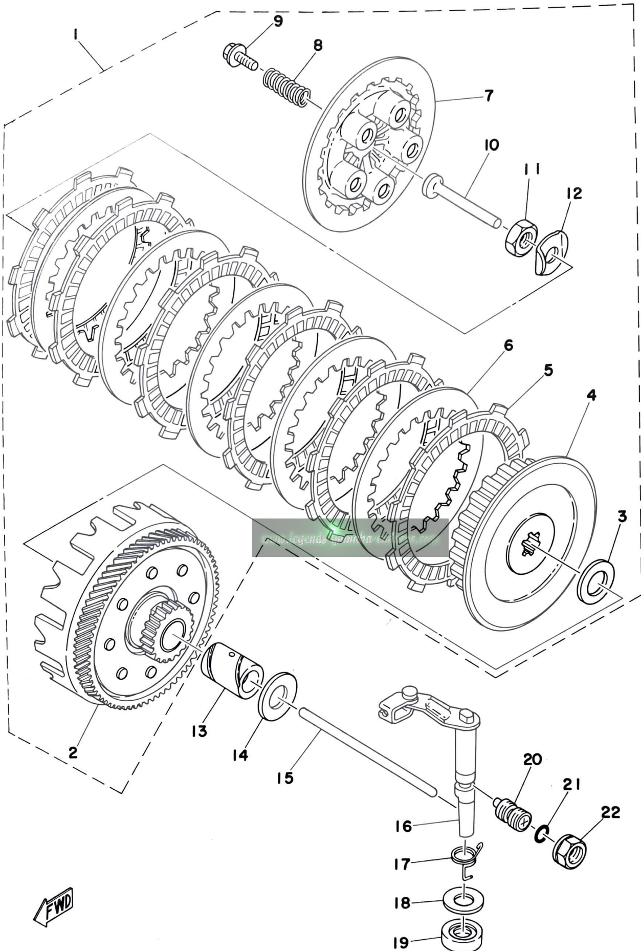
Fig. 4 CLUTCH
