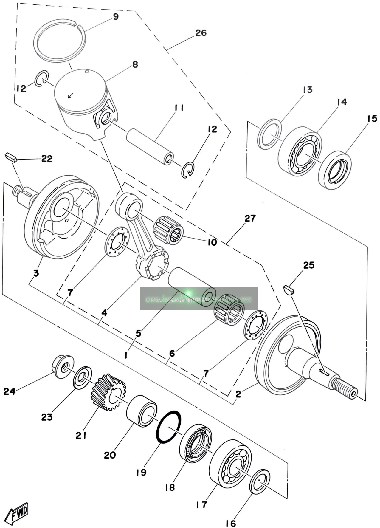
Fig. 3 CRANK · PISTON
