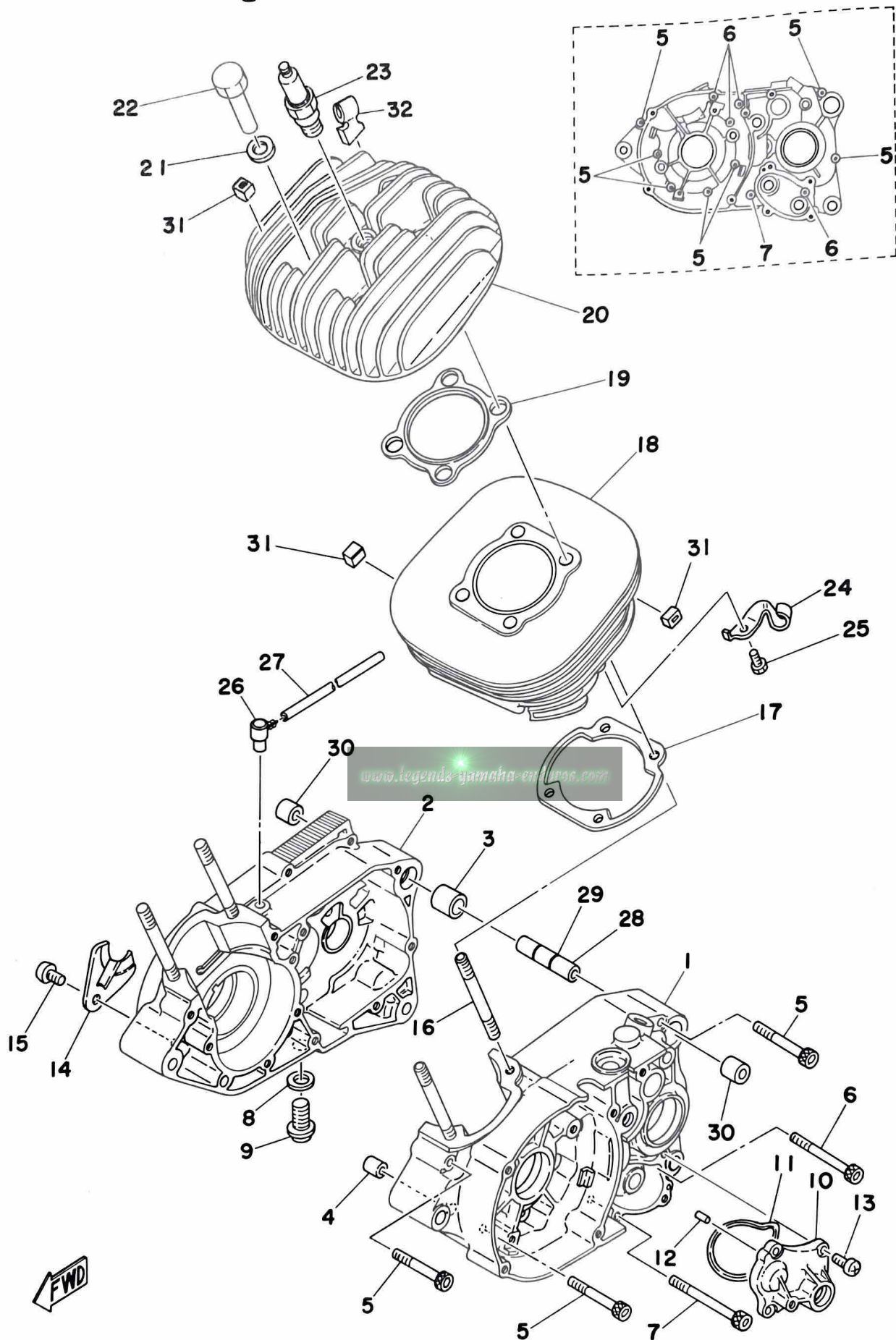
Fig. 1 CRANKCASE · CYLINDER
