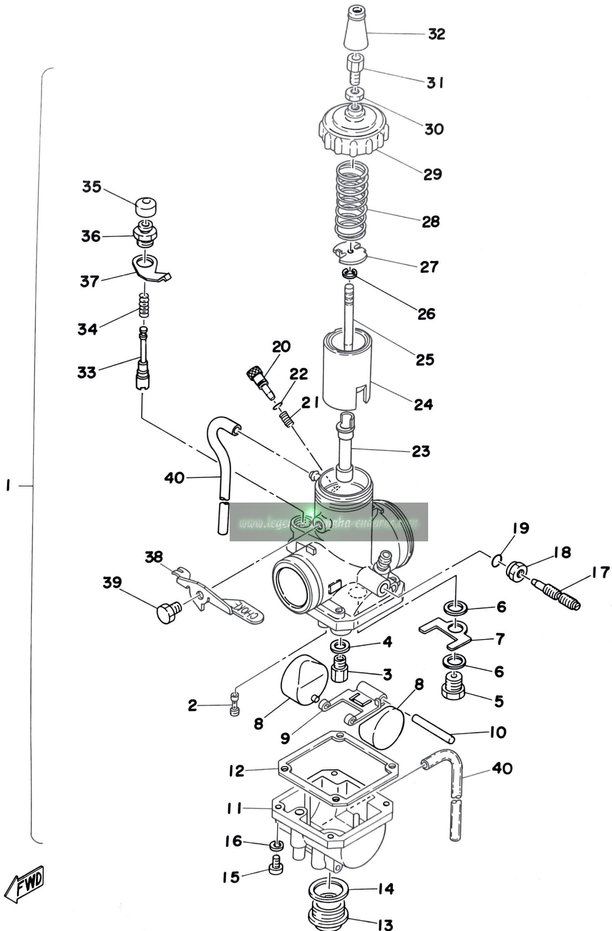
Fig. 10 CARBURETOR
