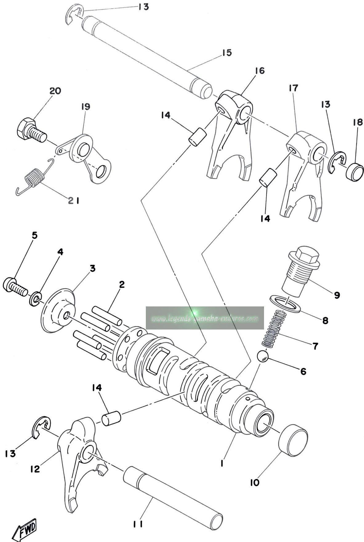
Fig. 6 SHIFTER 1
