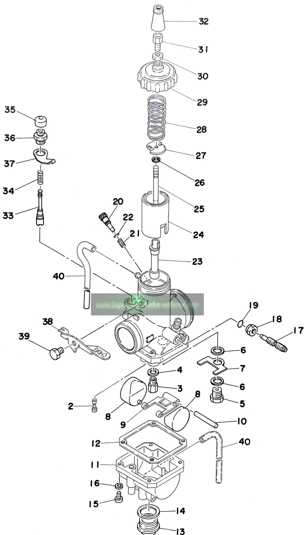
Fig. 10 CARBURETOR
