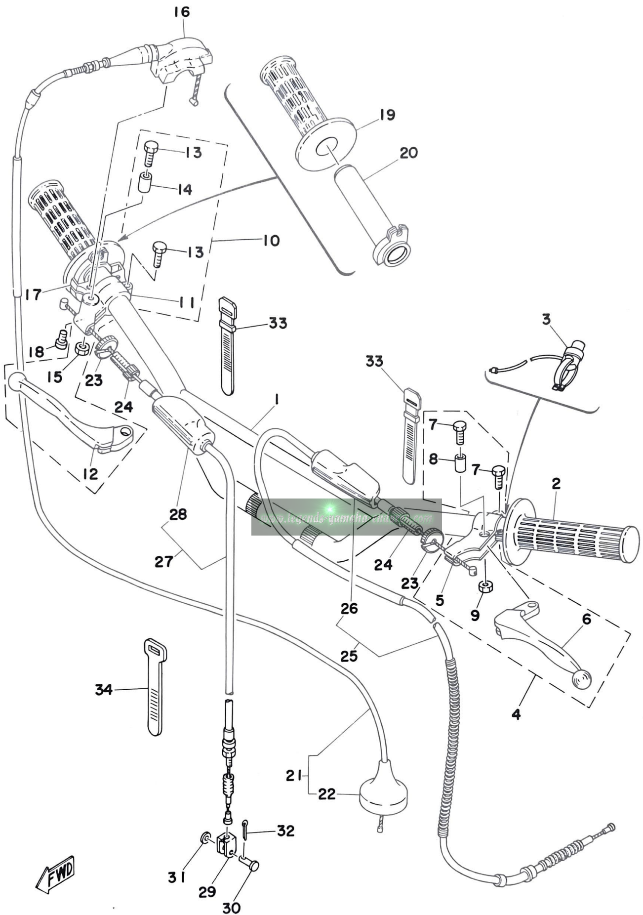
Fig. 19 HANDLE · WIRE
