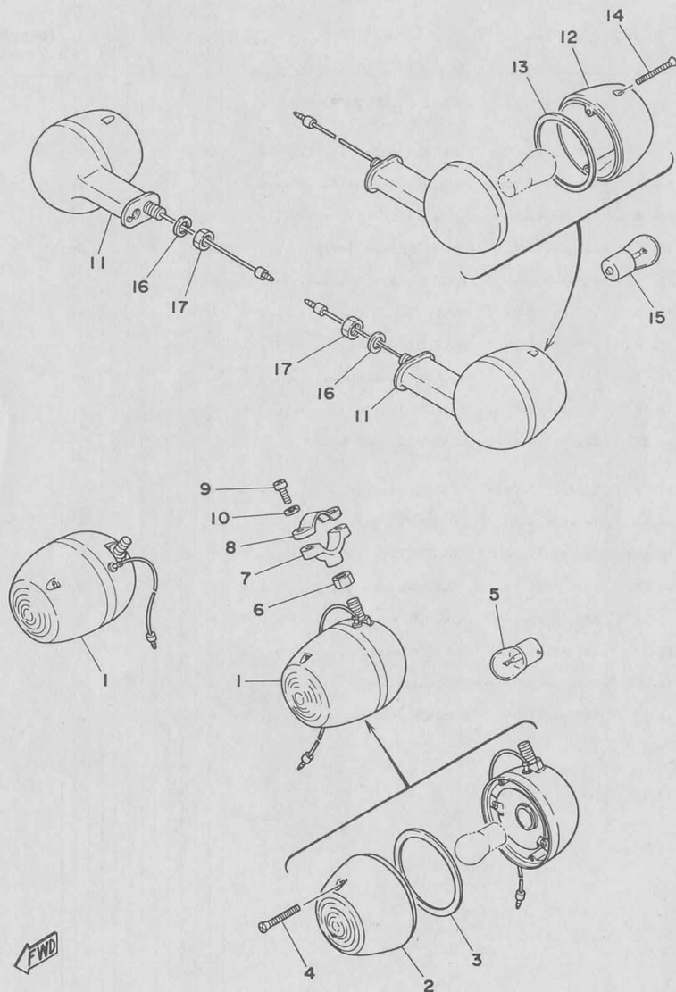
Fig. 33 FLASHER LAMP 2
