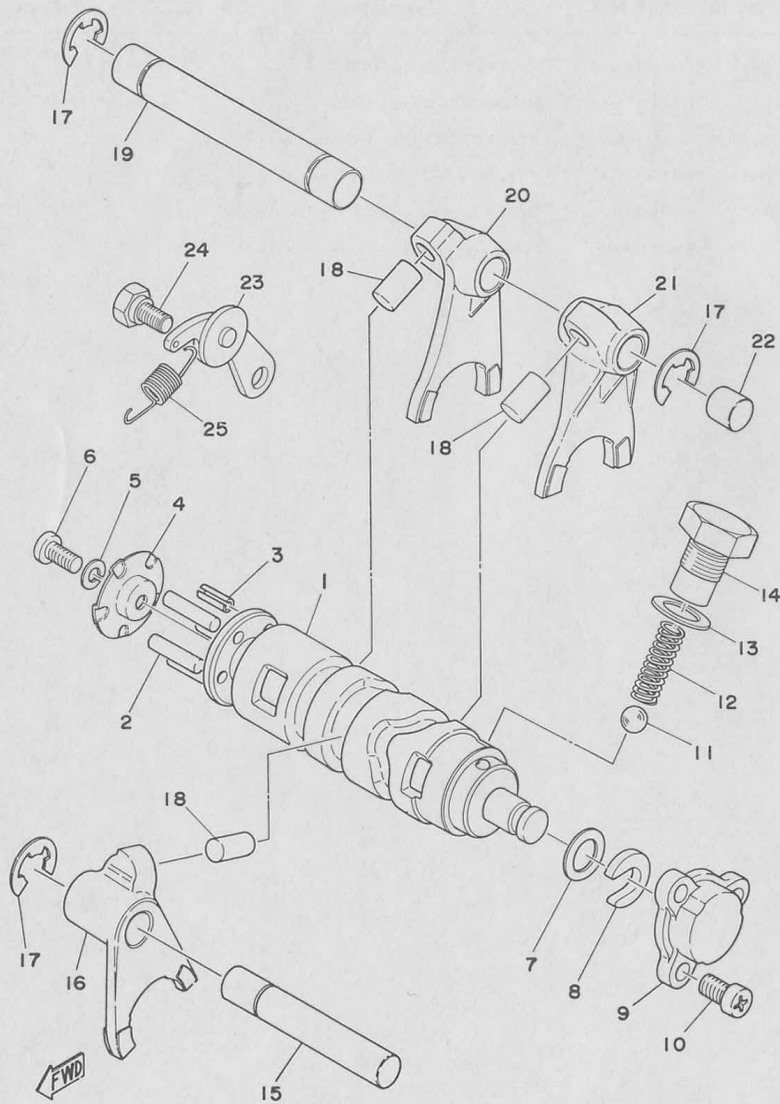
Fig. 6 SHIFTER 1
