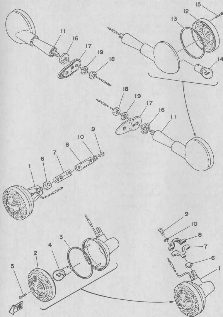
Fig. 32 FLASHER LAMP 1
