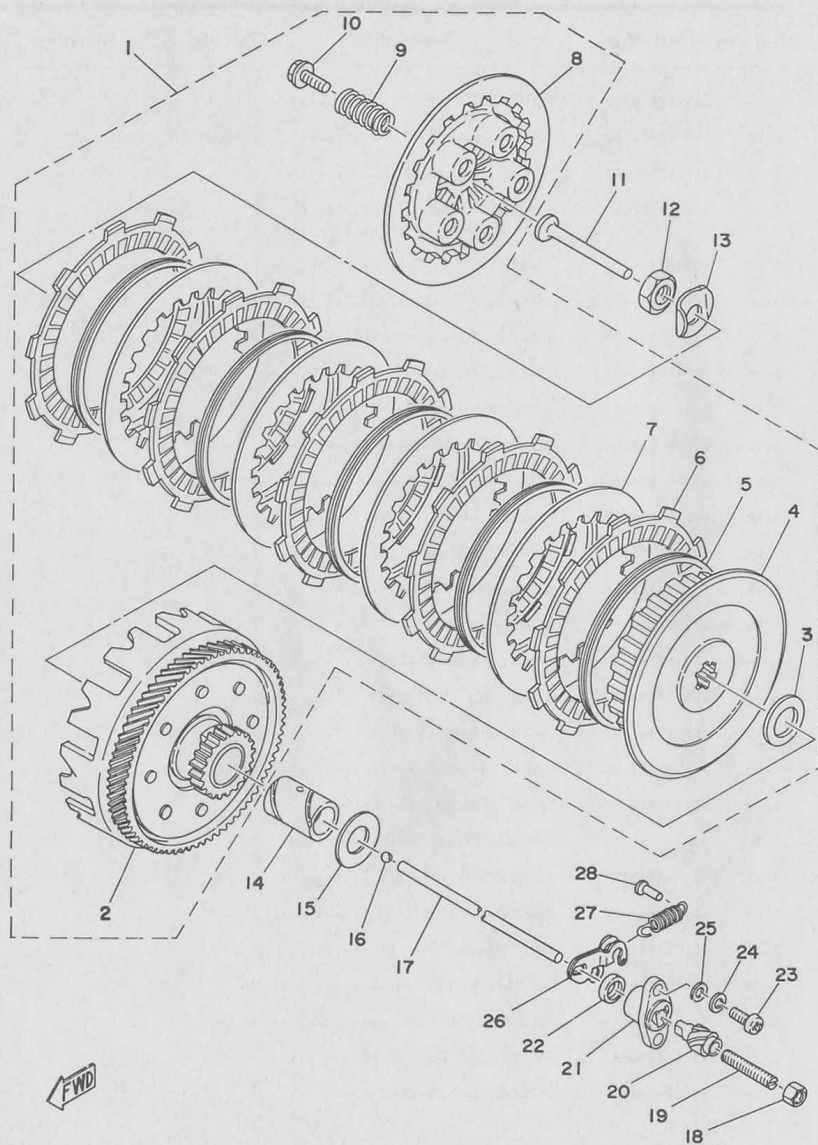
Fig. 4 CLUTCH
