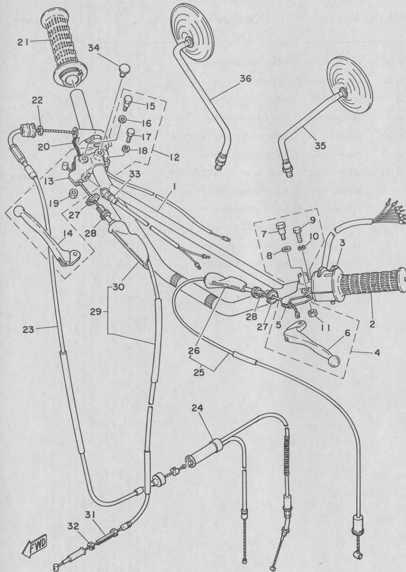
Fig. 21 HANDLE · WIRE
