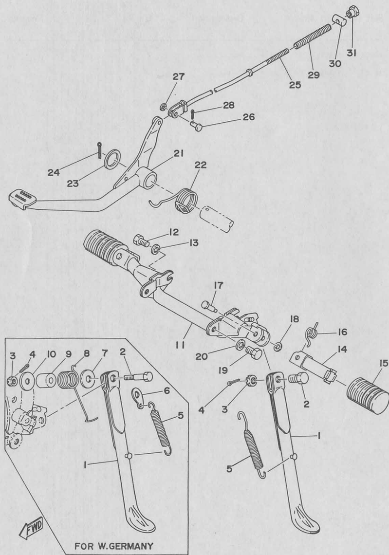
Fig. 17 STAND · FOOTREST · BRAKE PEDAL
