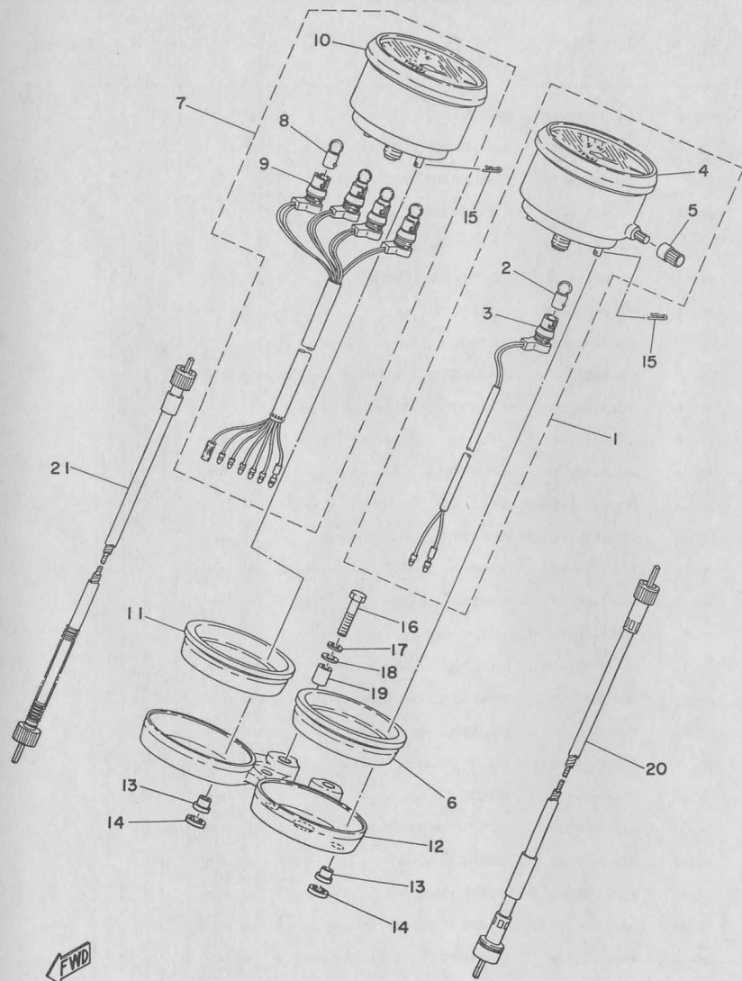
Fig. 29 SPEEDOMETER · TACHOMETER
