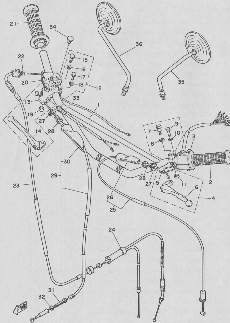
Fig. 21 HANDLE · WIRE
