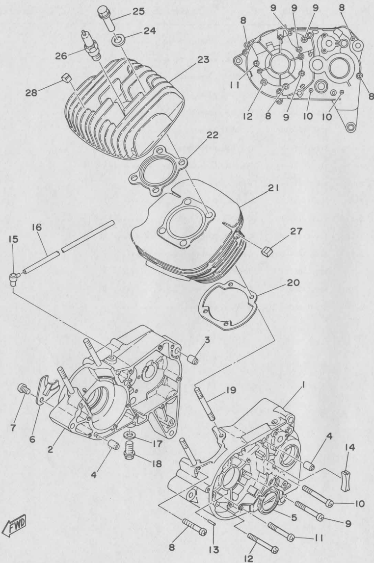
Fig. 1 CRANKCASE · CYLINDER
