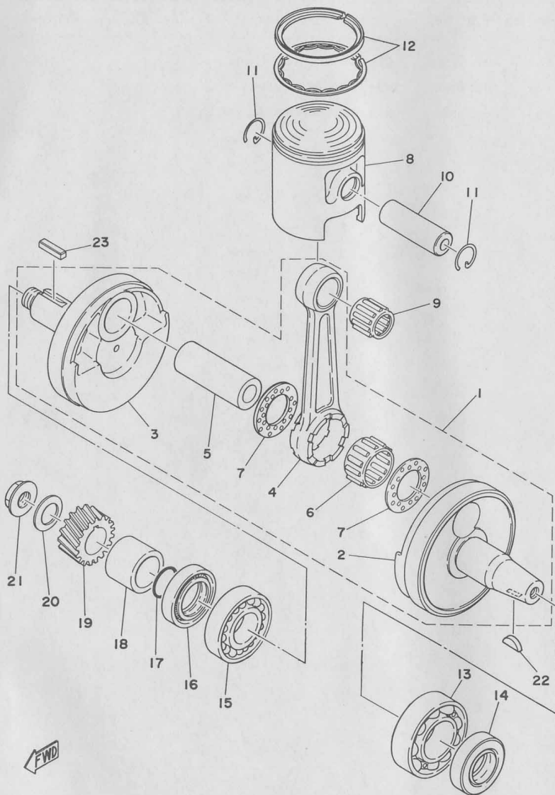
Fig. 3 CRANK · PISTON
