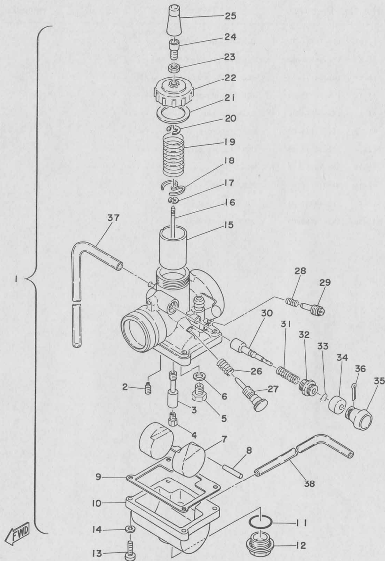
Fig. 11 CARBURETOR
