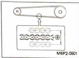
a Chain slack
