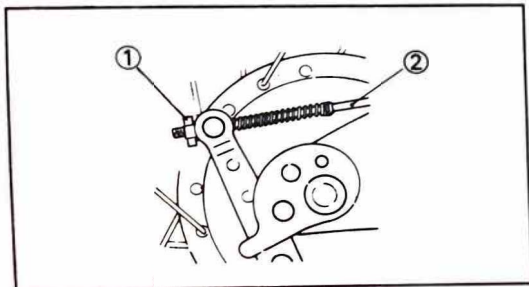
2. Brake rod
