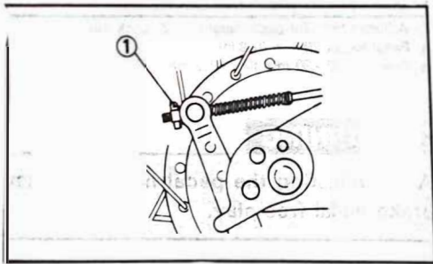
1. Adjuster
